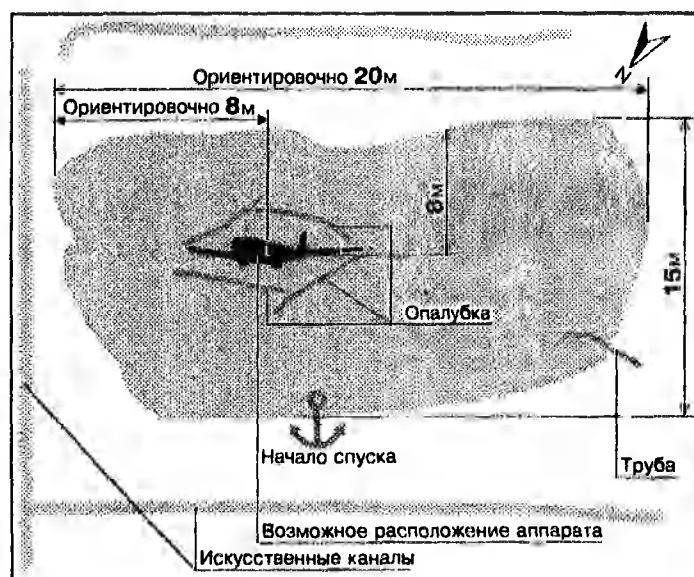
Схема извлечения из болота самолета «Нормандия-Неман».
