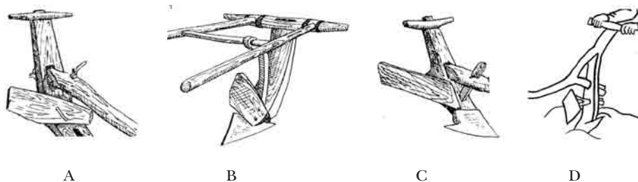
рис. 4.1. А — китайский плуг с фрески 630 г. 44 , В — сабан Уфимской губернии, С — «вятская соха», D — «казанский сабан» 45 .
